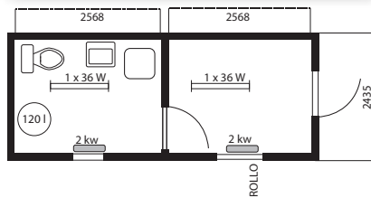
> Warmwasserbereiter 120 l
