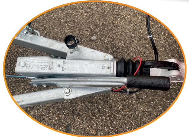
Mechanische Handbremse
