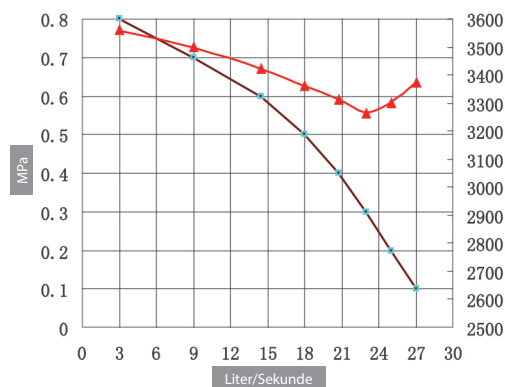
Leistungskurve
